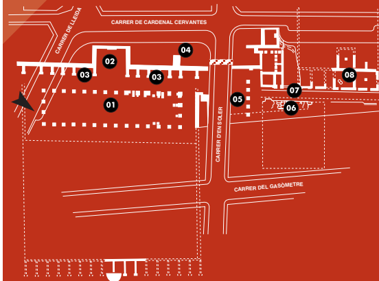
01 Basílica - Columnata de la nau central. 02 Cúria - Aedes Augusti . 03 Espais amb volta. 04 Cisterna de casa ( S. II aC). 05 Sala hipòstila. 06 Temple Capitolí. 07 Carrer. 08 Illa de cases.
