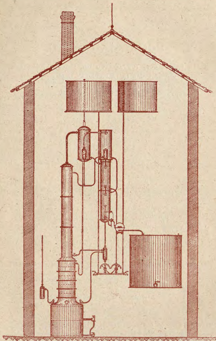
APARATO A FUEGO DIRECTO para la destilación de vinos produciendo alcoholes de 95 % 96 % con separación simultánea de cabezas y colas
