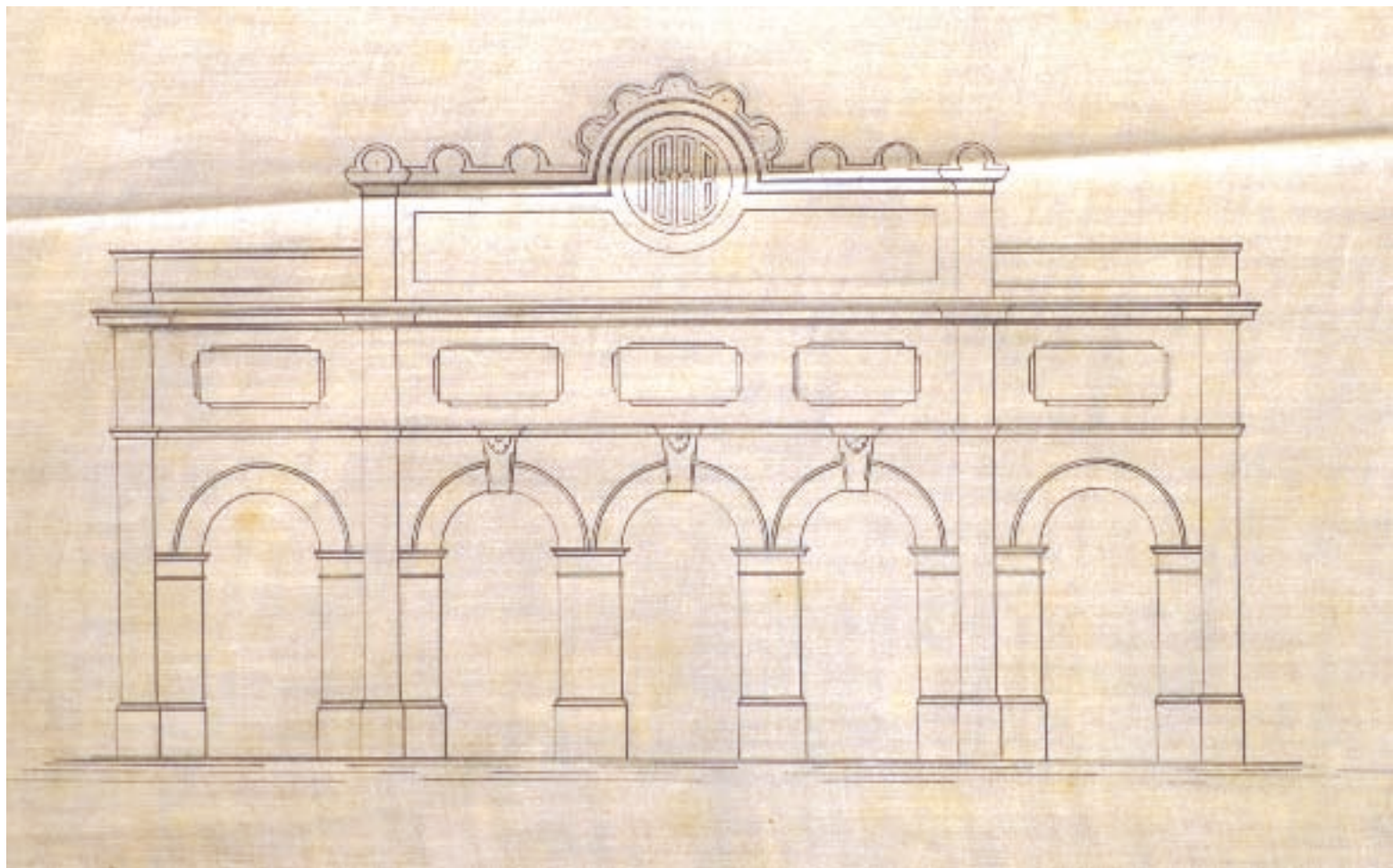
Projecte de reforma del Teatre Ateneu Tarraconense de la Classe Obrera. Fa- çana. Arquitecte: Ramon Salas Ricomà, 1888. Arxiu Salas.
