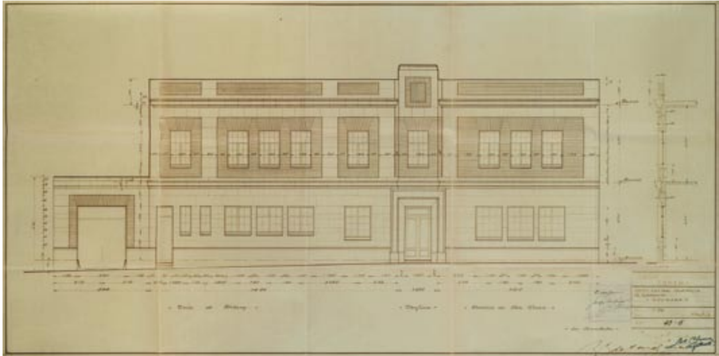
Plànol de Josep M. Pujol de la façana de l'edifici de la Central Telefònica, a la rambla del 14 d'Abril, xamfrà amb el carrer Fortuny, any 1933. AMT, Eixample 16/34.
