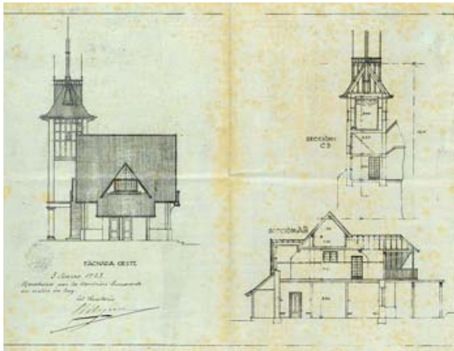
Projecte del pavelló que es va construir en el camp d'esports de l'Avinguda Catalunya, maig 1924. AMT, P 4054.
